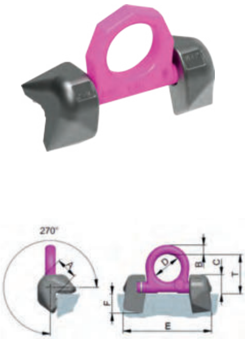
Ringbock schweisssbar für 90°-Kanten Allseitig belastbar, leichte und einfache Schweissmontage, bis 270° schwenkbar. Eine geschützt liegende Feder hält den Aufhängebügel in jeder gewünschten Lage.
