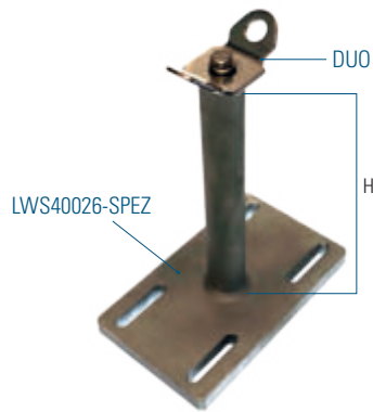
Bestehend aus Platte mit 4 Schlitzten und 4 Fasen, feuerverzinkt, mit 1x Innengewinde M16 und 4x Innengewinde M12.
