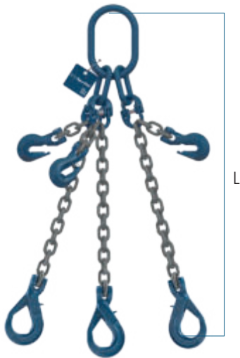
3-Strang-EXOSET®-Kettengehänge mit Ovalring, verkürzbar, mit selbstschliessendem Sicherheitshaken CRFX oder mit Lasthaken mit Sicherung CBX
