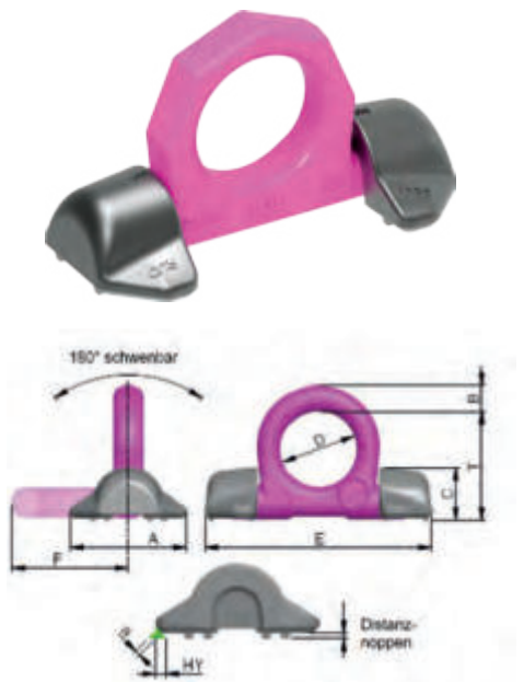
Ringbock schweisssbar Allseitig belastbar, leichte und einfache Schweissmontage.
